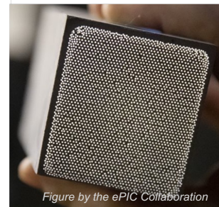
Forward EM Calorimeter
